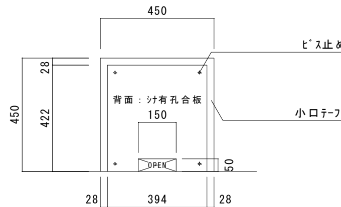
【 背面図 】
