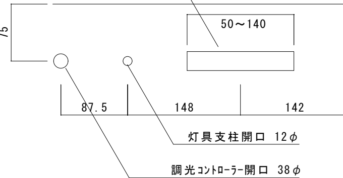
【 開口詳細図 S=1/5 】
